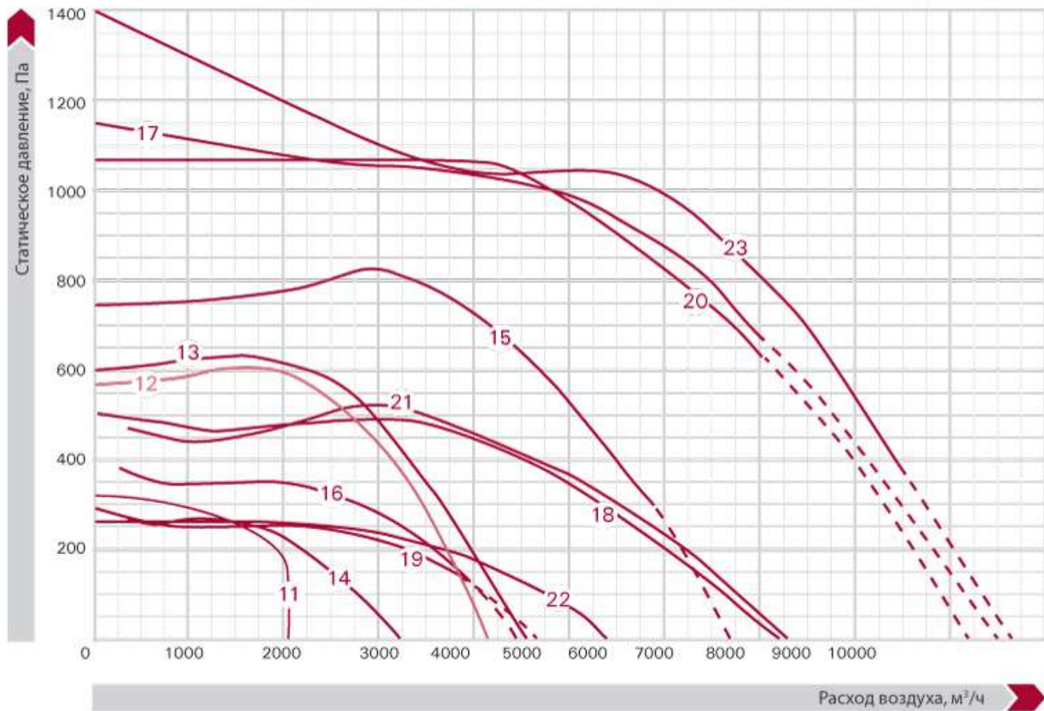
Аэродинамические характеристики вентиляторов сечением от 600x350 до 1000x500
